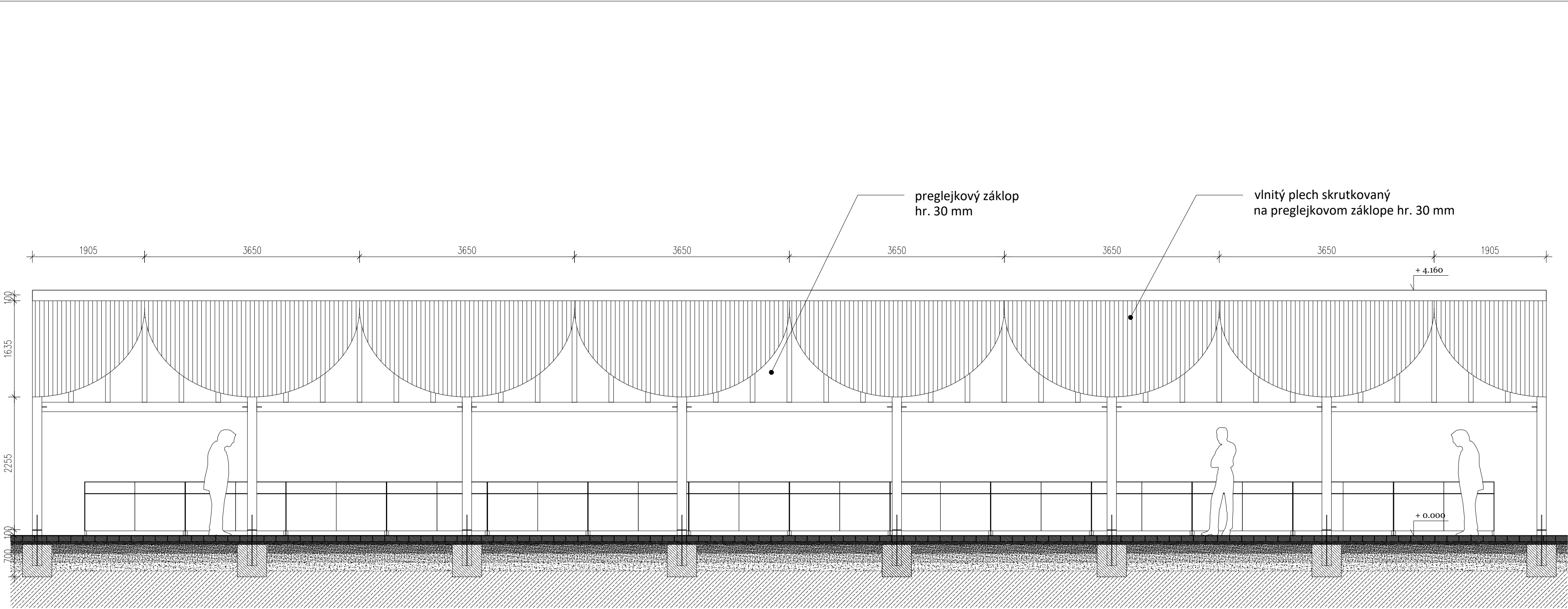
POHĽAD SEVEROVÝCHODNÝ (s oblúkmi)
