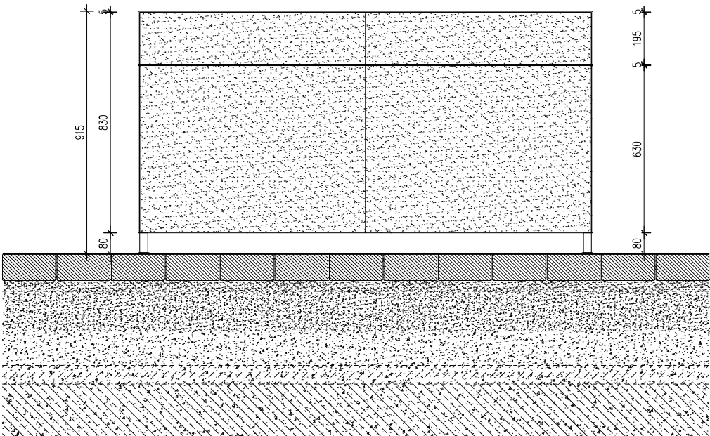
pohľad zo strany kupujúceho
