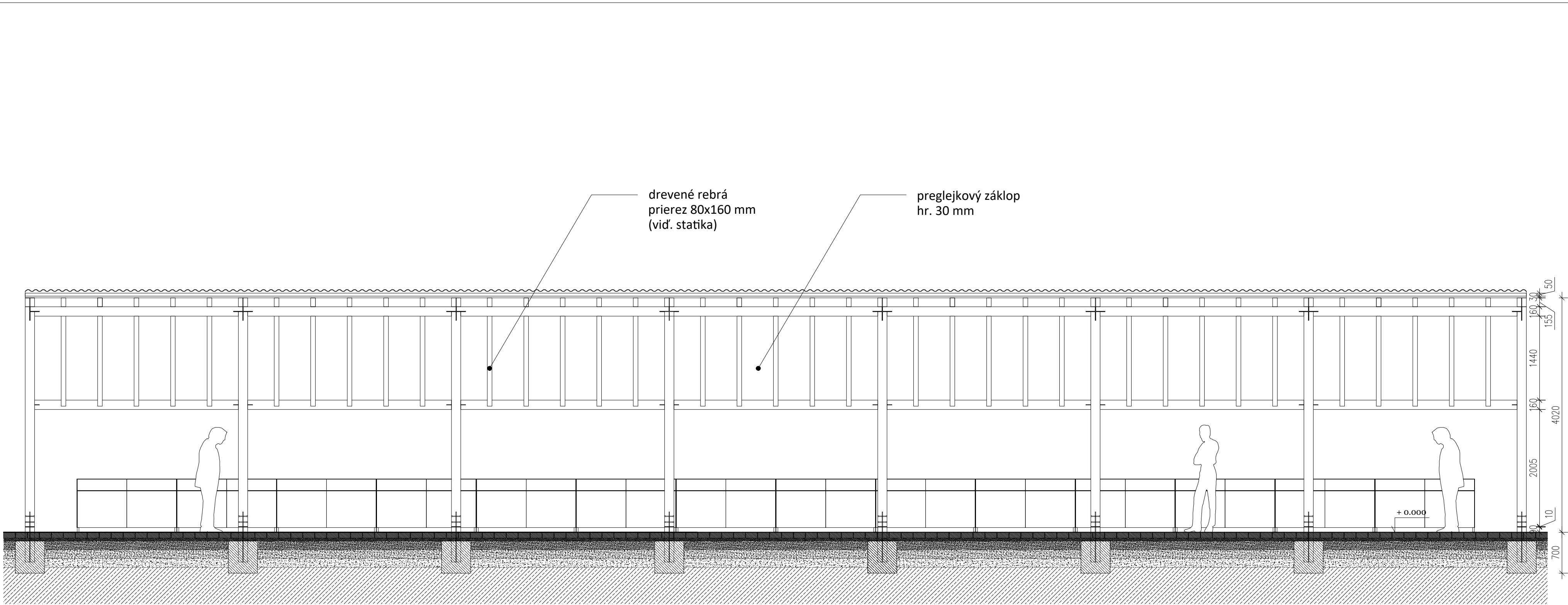
POHĽAD SEVEROVÝCHODNÝ (bez oblúkov)
