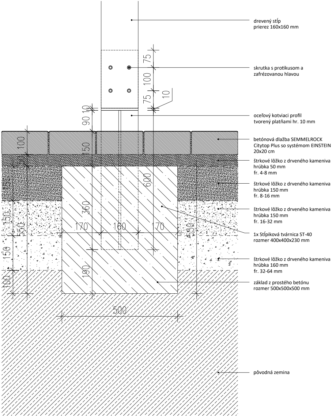
rezopohľad
