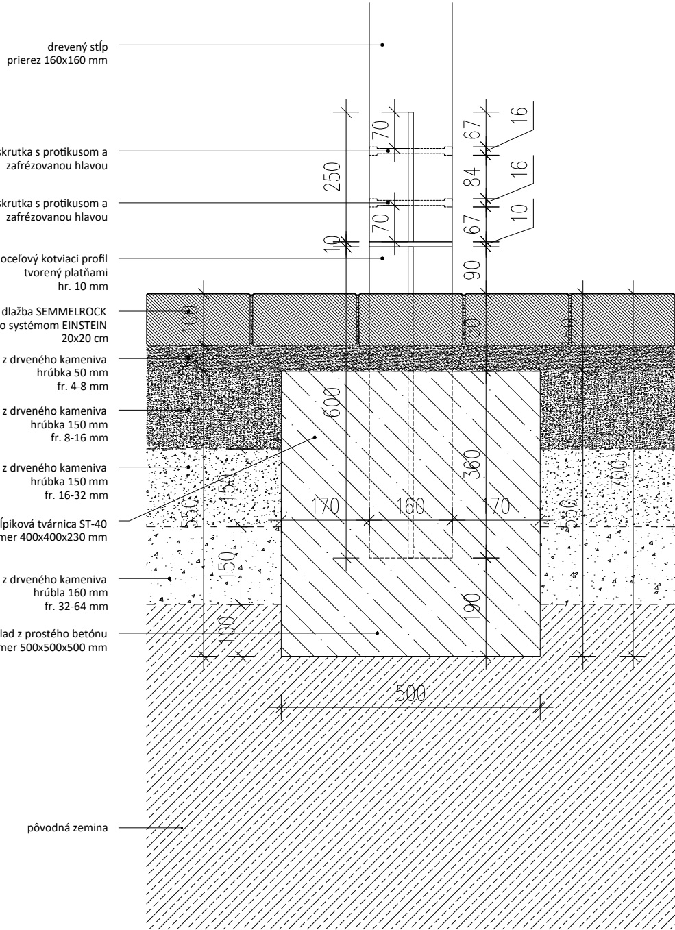
rezopohľad
